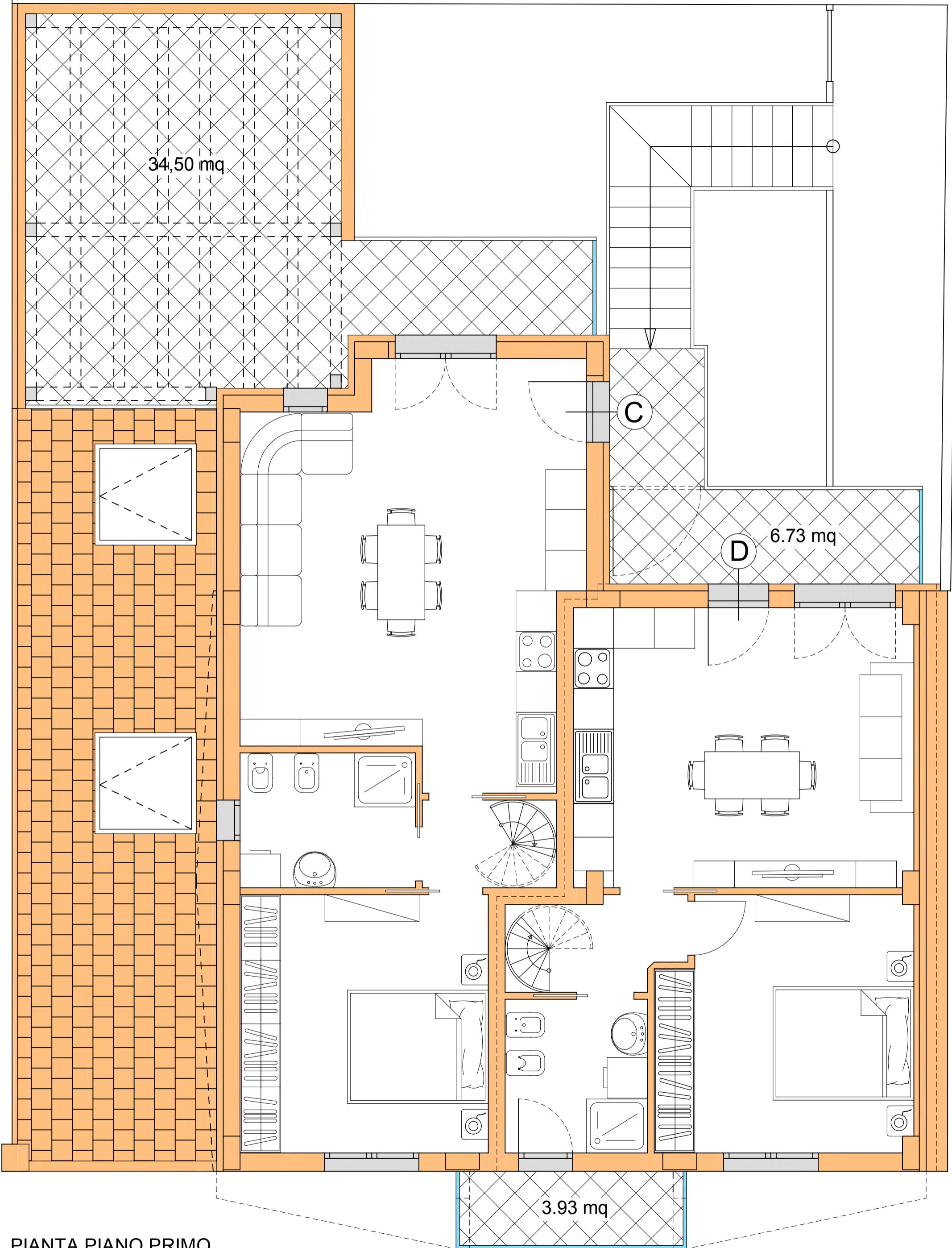
PIANTA PIANO PRIMO SCALA 1:50
